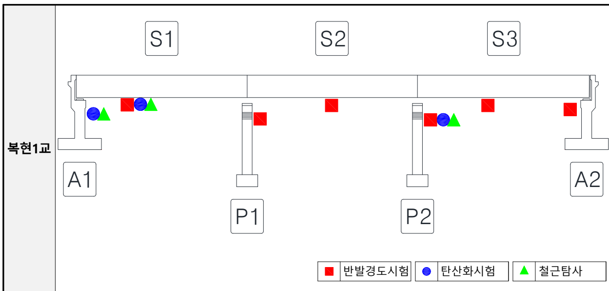
[그림 4.1.2] 비파괴시험 위치도
